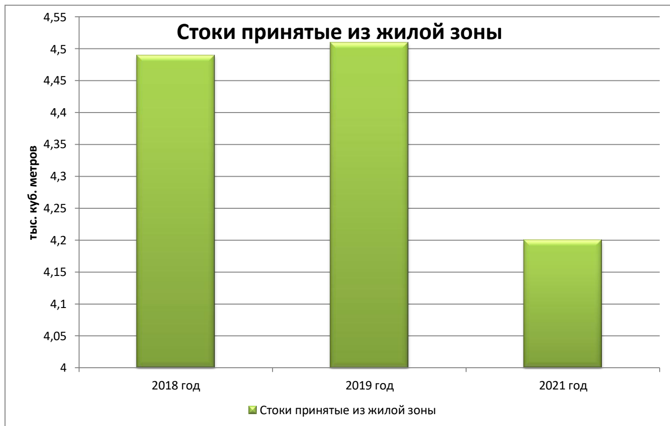
Диаграмма 3 – Динамика поступления сточных вод с систему централизованного водоотведения по зонам за 2018-2021 год
